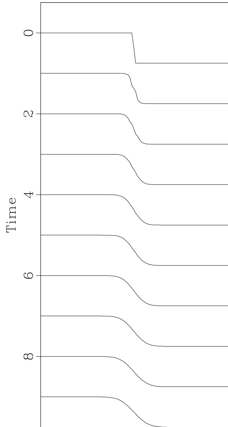
Implicit, a=2
