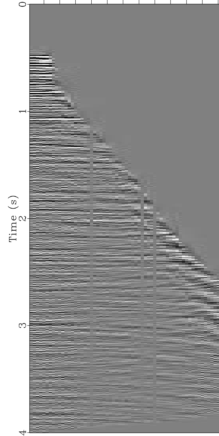
NMO
