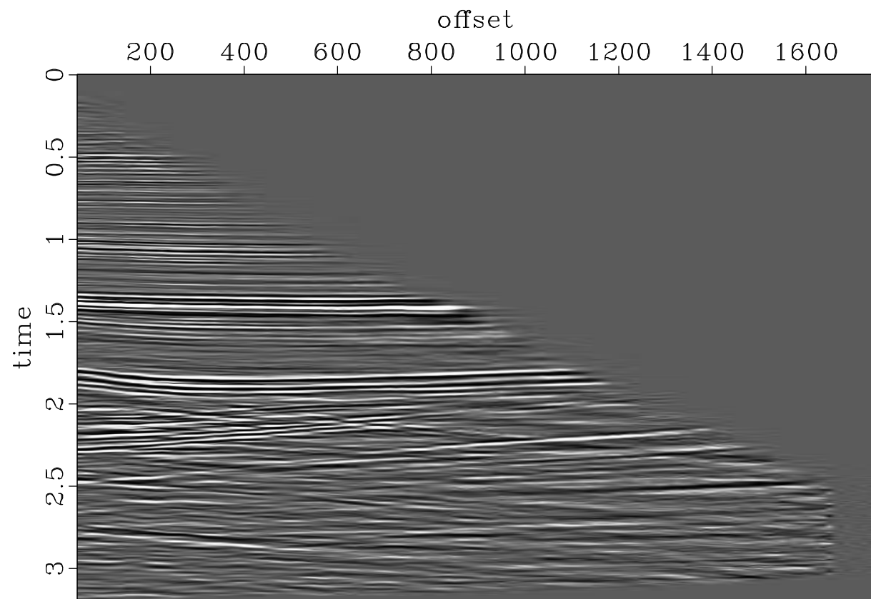
(\text{shot1} + \text{shot3}) / 2
