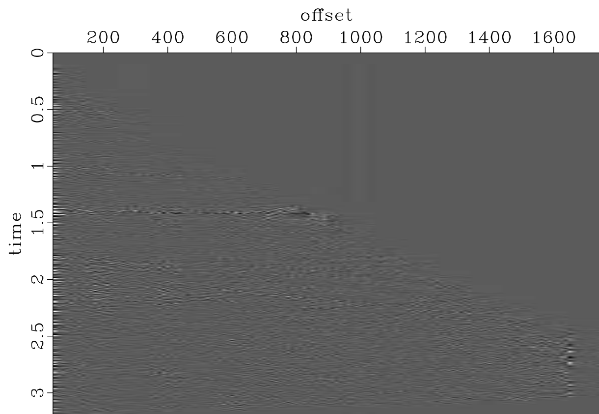
error
