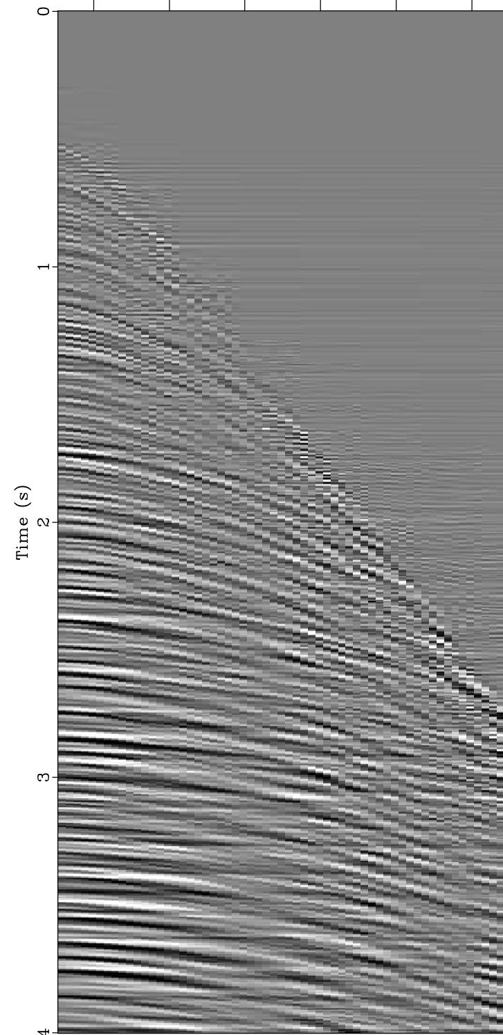
Adjoint Hyperbolic Radon Transform
