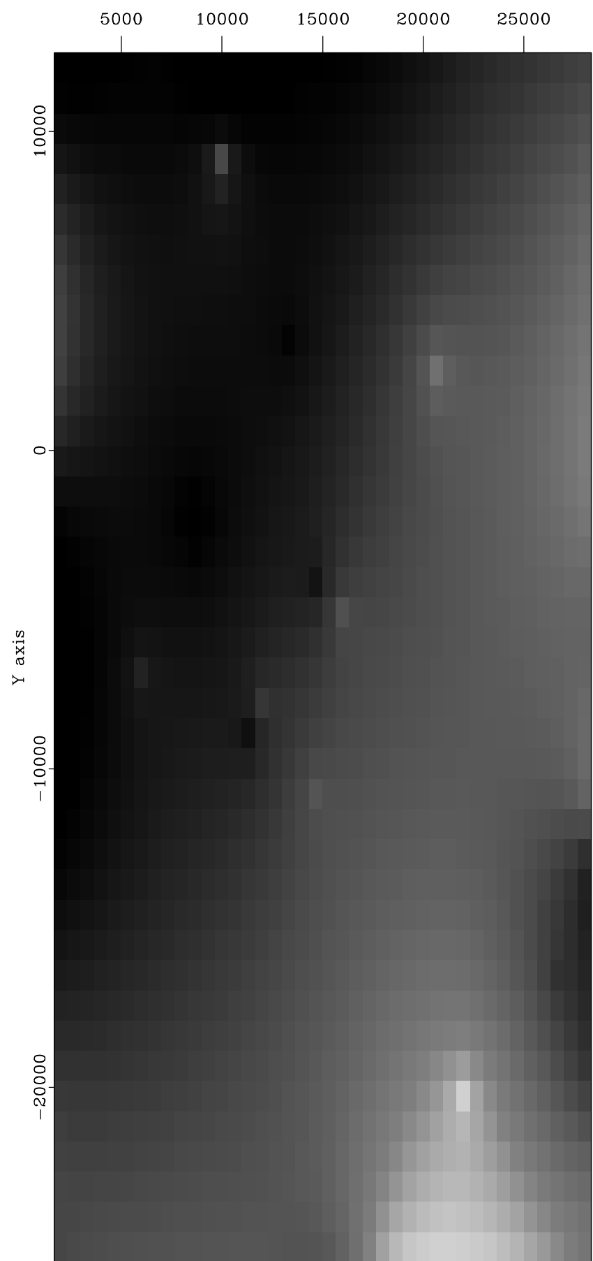
Gradient Map - Seismic
